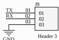
Debug_UART
