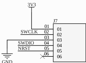
Header 6
